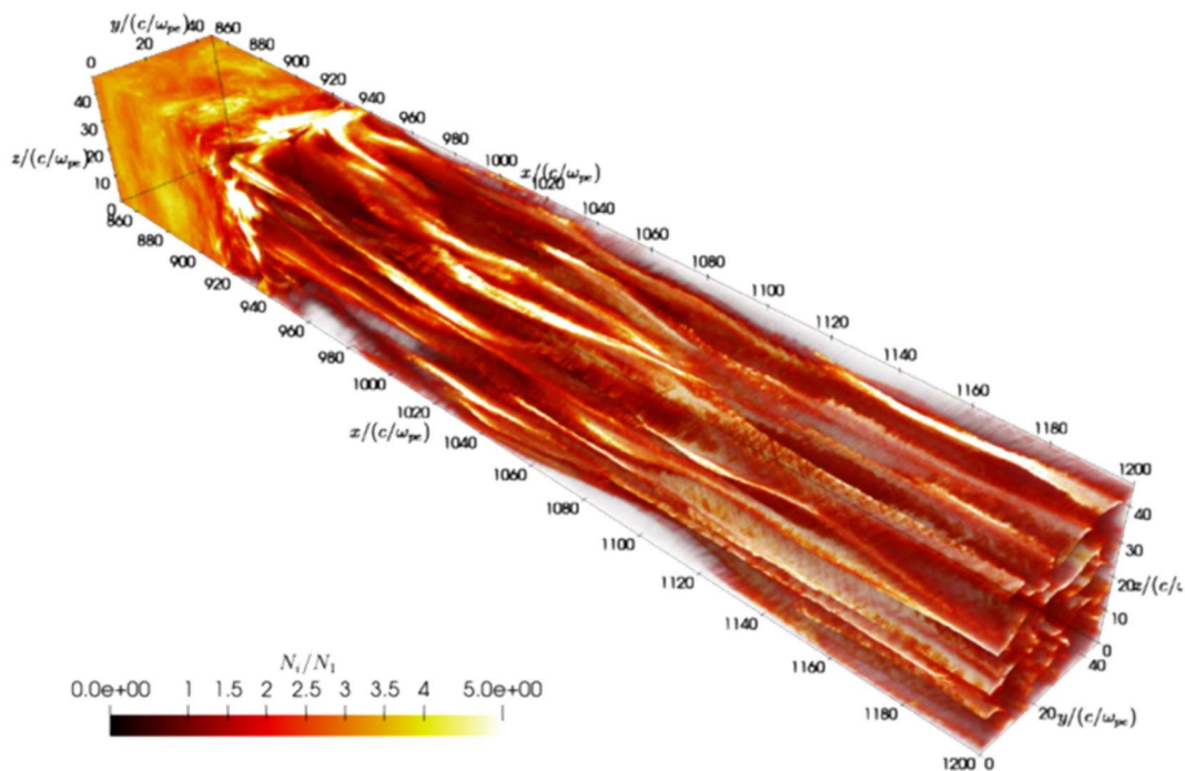
図：3次元PICシミュレーションによる相対論的衝撃波の密度構造
