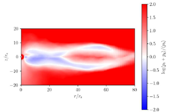
図：増光時の活動銀河中心核降着流の低解像度輻射磁気流体シミュレーション結果（五十嵐太一博士論文、計算は国立天文台の XC50 を用いて実施）。カラーは（ガス圧+輻射圧）/磁気圧。長さの単位はシュバルツシルト半径。
